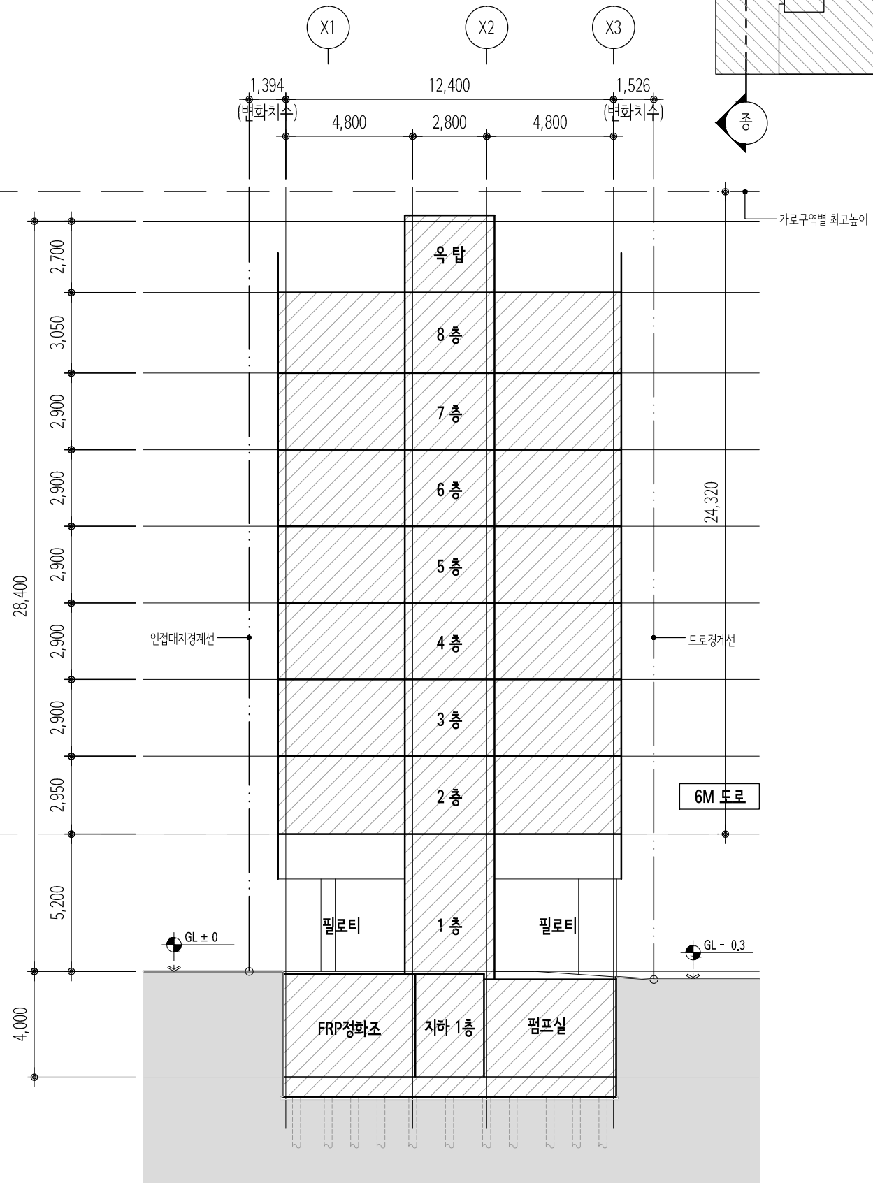
2 A 대지 "횡" 단면도 축척 : 1 / 200
