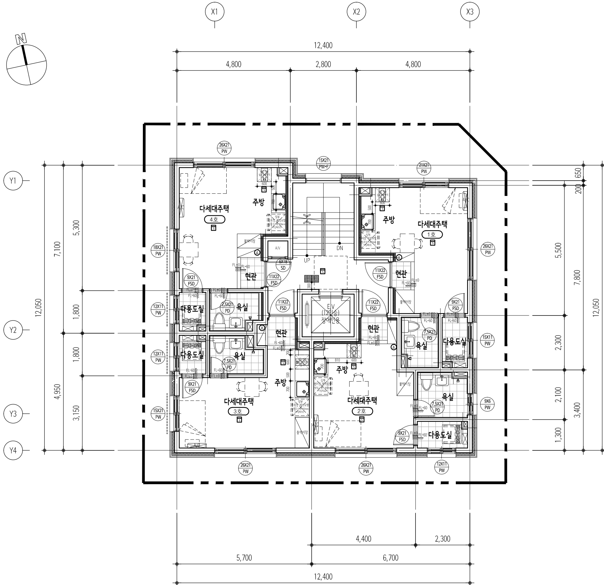
1 A 지상2층 평면도 (다세대주택) 축척: 1 / 100
