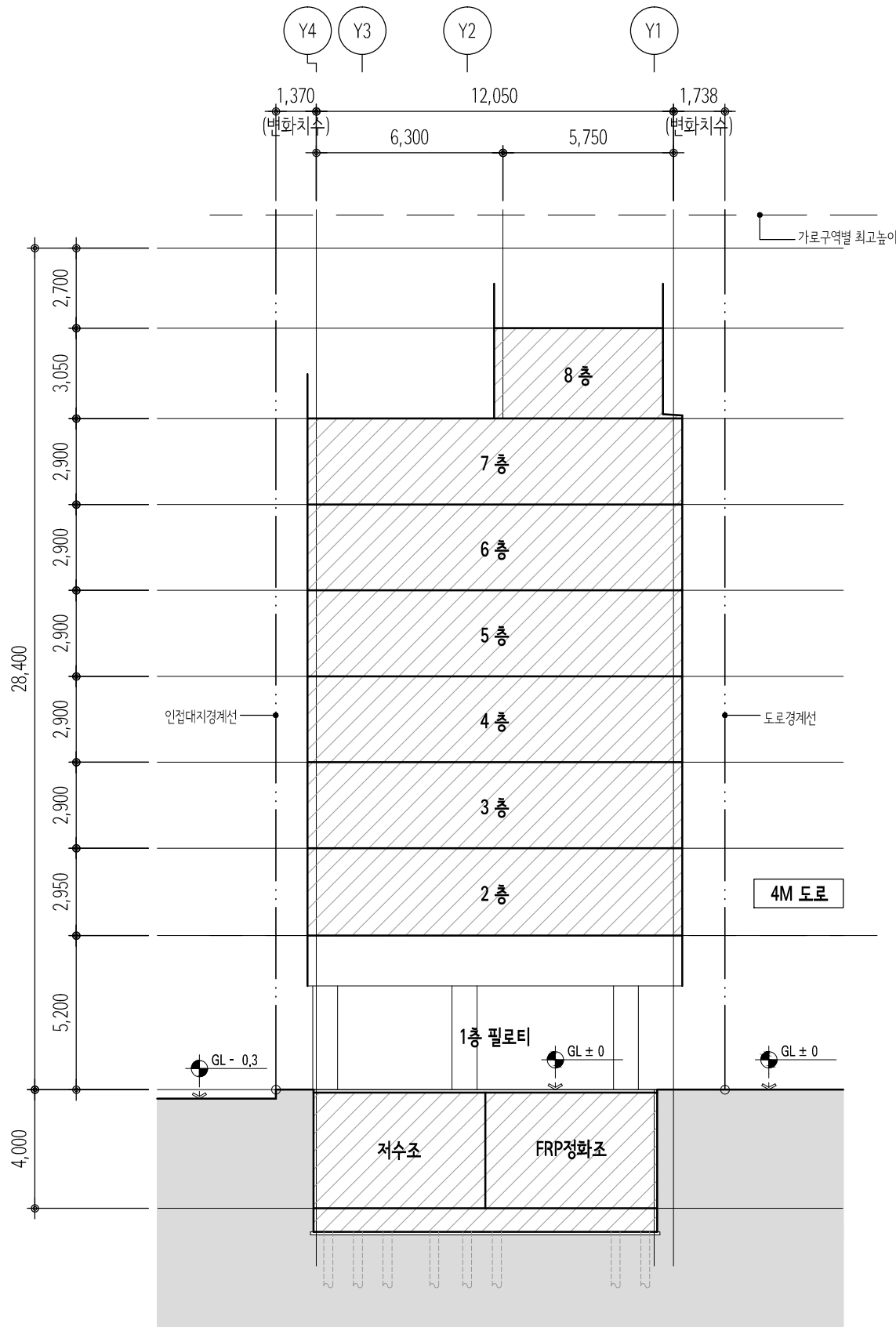
1 A 대지 "종" 단면도 축척 : 1 / 200
